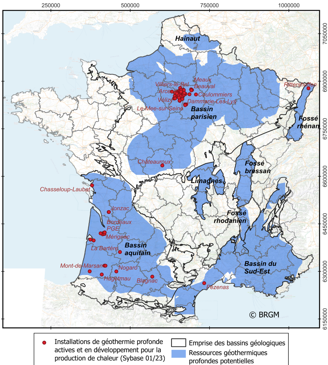
Figure 3 : aquifères profonds en France métropolitaine. Source : BRGM.
