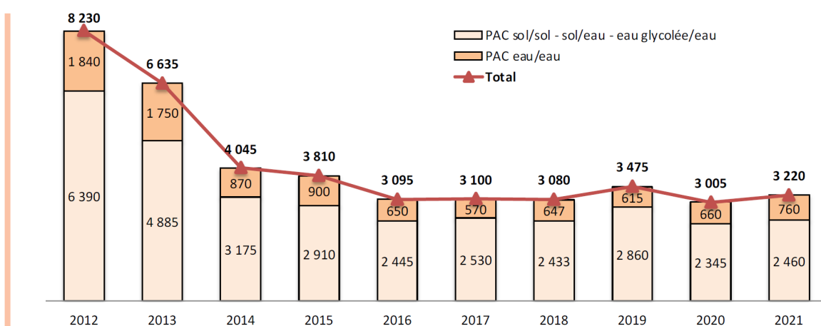
Figure 2 : évolution du nombre de pompes à chaleur géothermiques vendues en France de 2012 à 2021. Source : Observ'ER.
