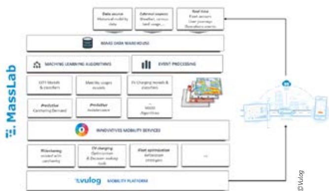
Structure logicielle Maaslab
