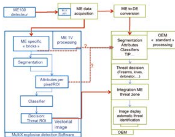
Logiciel ME de détection d'explosifs (bloc bleu) : architecture/ fonctions et interfaces avec le logiciel OEM du scanner (bloc vert).
