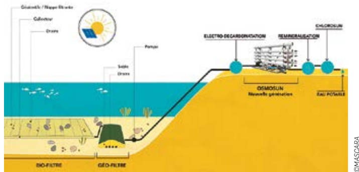
Procédé ECODESS pour le dessalement d'eau de mer
