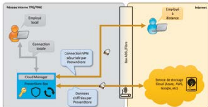
Mise en œuvre de la solution ProvenStore
